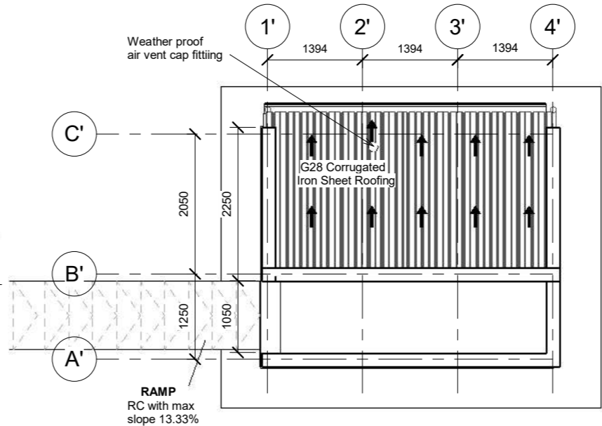
2 ROOF PLAN 1 : 50
