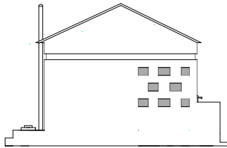
RIGHT ELEVATION
